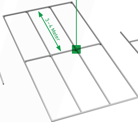
ALUFIX Unterkonstruktion mit Stossver- bund
